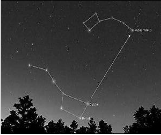
Şekil 8. Kuzey/kutup yıldızı.
