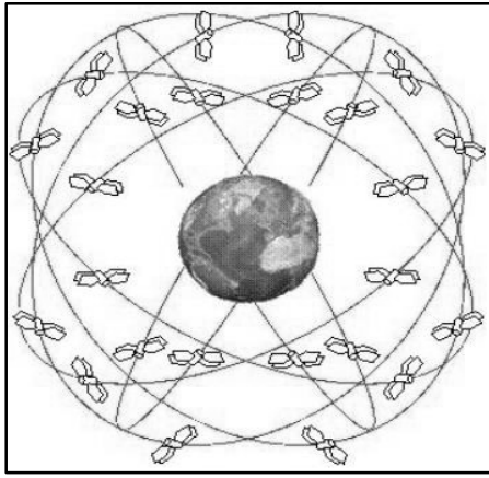
Şekil 4. GPS/GNSS uyduları.
